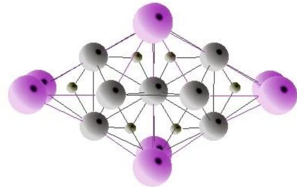
\text{LaNi}_5\text{H}_6
